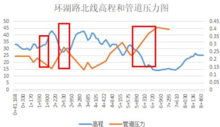
图 7-14 环湖路北线高程和管道压力差图（红框为爆漏频繁管段）
