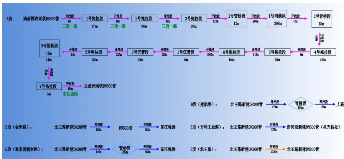
图 7-21 北海产业园区管道路由及管线布置图
