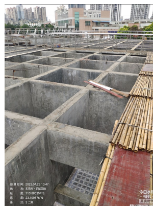
图 8-10 黄洲水厂网格絮凝池
