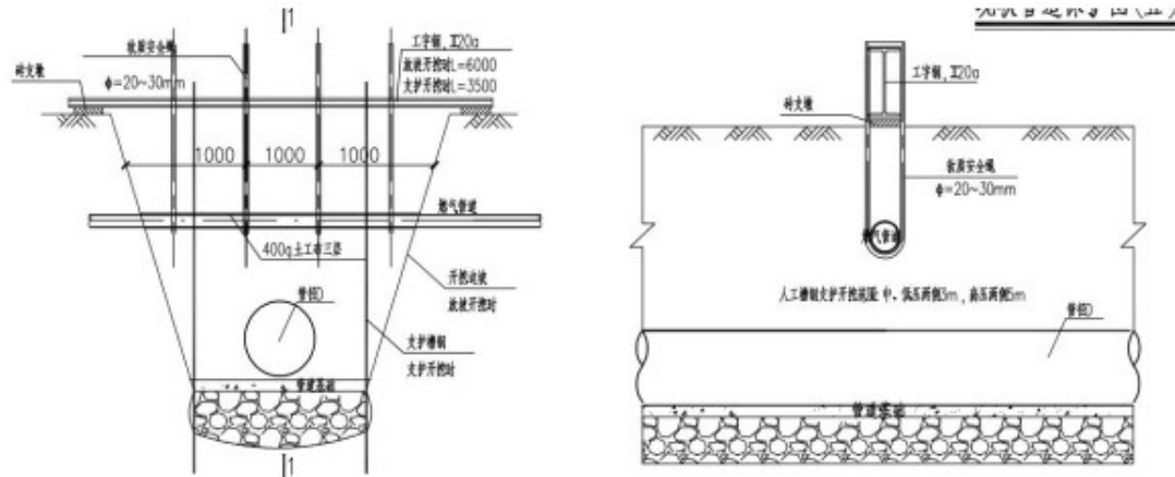
图 8-19 燃气管道保护大样图
